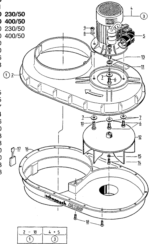
Gehäuse mit Motor 7503 1000
